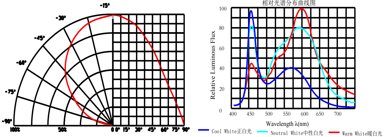
Wavelength Characteristics T_a=25^\circ\text{C} 相对光谱分布曲线图
